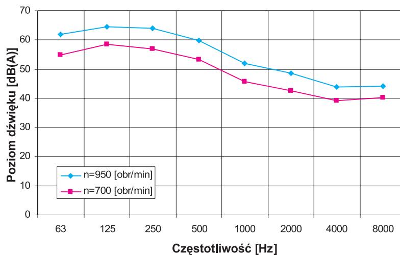
Charakterystyka akustyczna wentylatora WDc 40 z tłumikiem PTH 40 lub z podstawą tłumiącą PPT 40 (na wlocie w odległości 1m).
