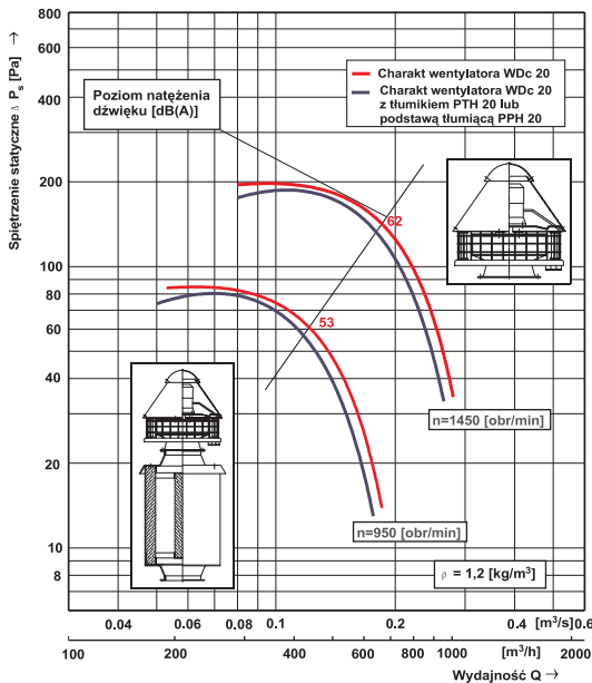
Charakterystyka przepływowa wentylatora dachowego WDC 20 z tłumikiem lub z podstawą tłumiącą
