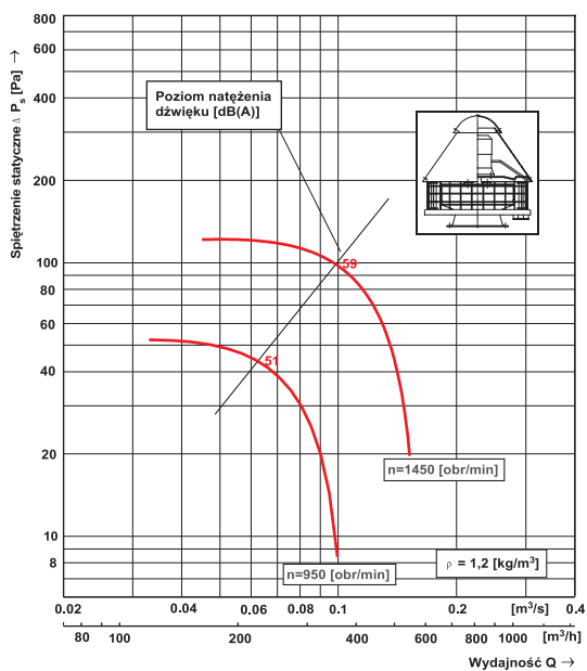
Charakterystyka przepływowa wentylatora dachowego WDc 16
