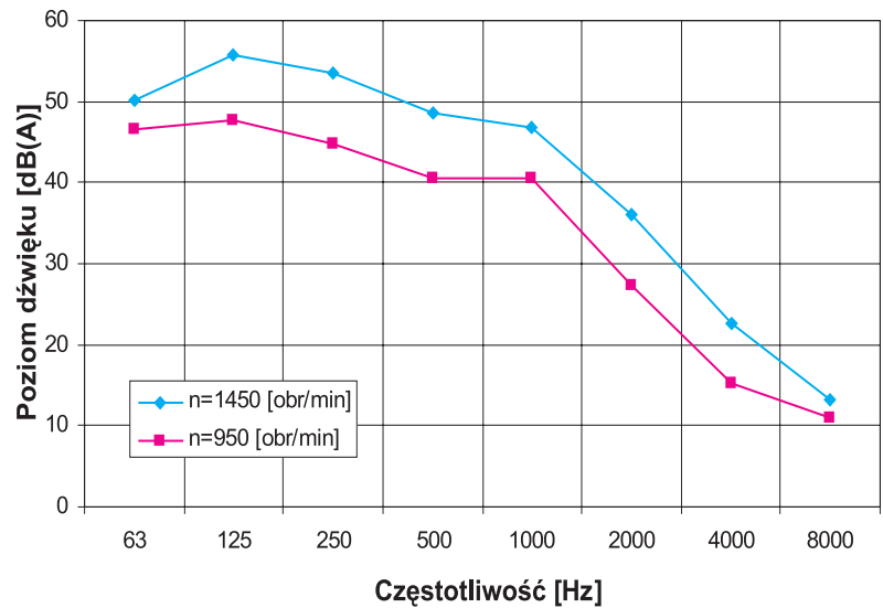
Charakterystyka akustyczna wentylatora WDC 20 z tłumikiem PTH 20 lub z podstawą tłumiącą PPT 20 (na wlocie w odległości 1m).
