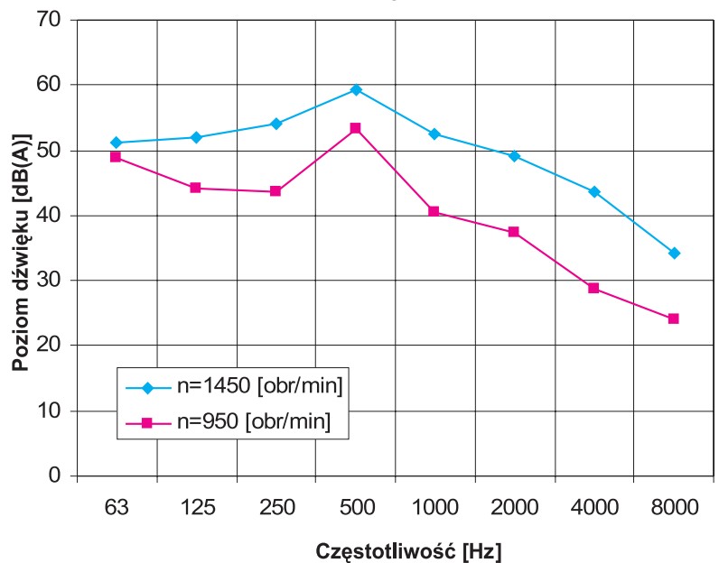
Charakterystyka akustyczna wentylatora WDc 16 (na wlocie w odległości 1m)
