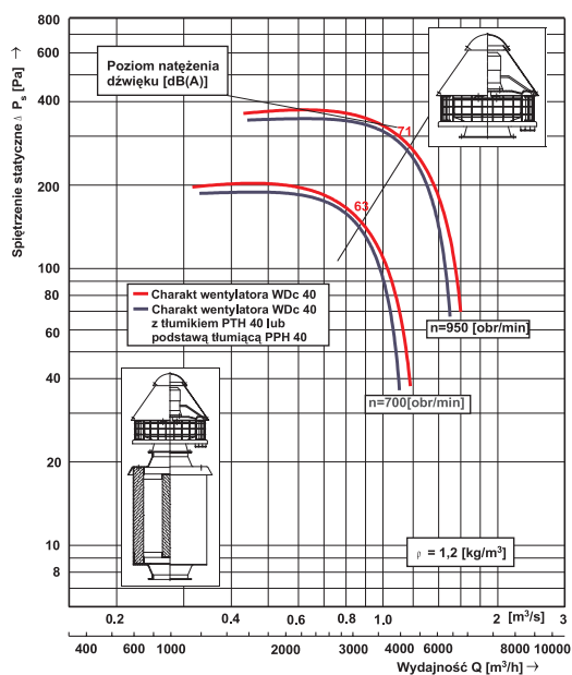
Charakterystyka przepływowa wentylatora dachowego WDc 40 z tłumikiem lub z podstawą tłumiącą
