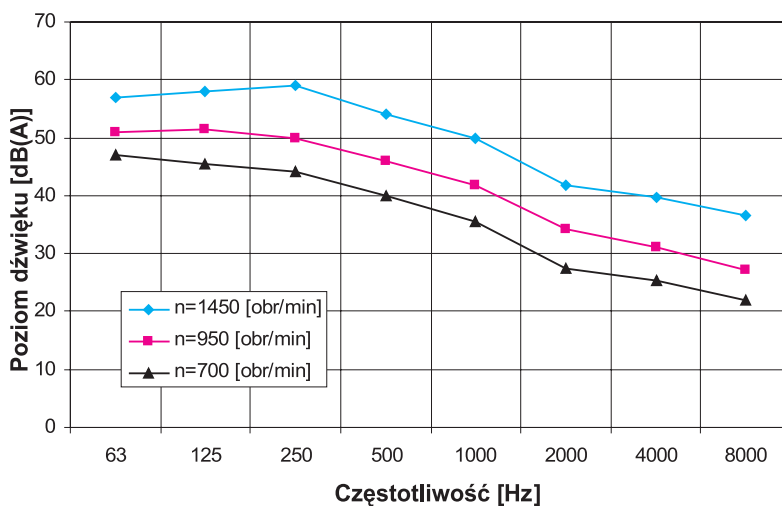
Charakterystyka akustyczna wentylatora WDC 31,5 z tłumikiem PTH 31,5 lub z podstawą tłumiącą PPT 31,5 (na wlocie w odległości 1m).
