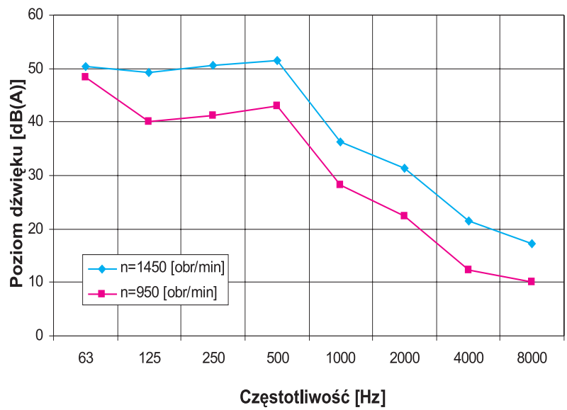
Charakterystyka akustyczna wentylatora WDC 16 z tłumikiem PTH 16 lub z podstawą tłumiącą PPT 16 (na wlocie w odległości 1m).
