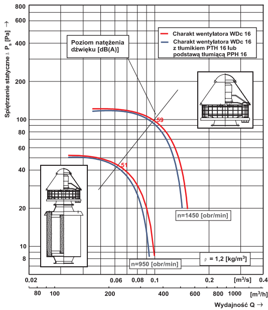
Charakterystyka przepływowa wentylatora dachowego WDC 16 z tłumikiem lub z podstawą tłumiącą
