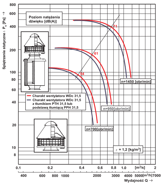
Charakterystyka przepływowa wentylatora dachowego WDC 31,5 z tłumikiem lub z podstawą tłumiącą
