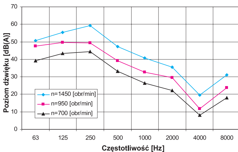
Charakterystyka akustyczna wentylatora WDC 25 z tłumikiem PTH 25 lub z podstawą tłumiącą PPT 25 (na wlocie w odległości 1m).
