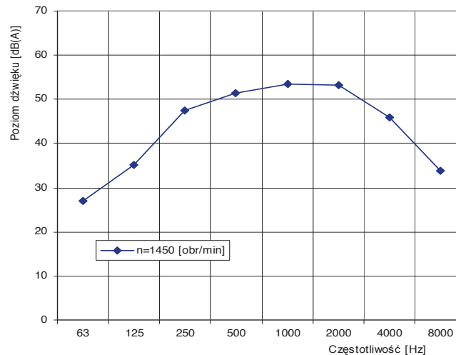
Charakterystyka akustyczna wentylatora dachowego WDC/s 20-Ex (na wlocie w odległości 1m)
