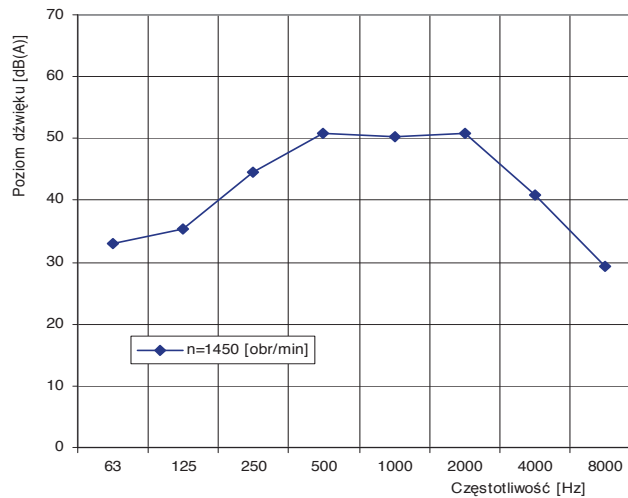
Charakterystyka akustyczna wentylatora dachowego WDC/s 16-Ex (na wlocie w odległości 1m)
