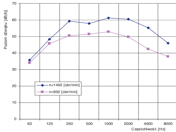
Charakterystyka akustyczna wentylatora dachowego WDC/s 31,5-Ex (na wlocie w odległości 1m)
