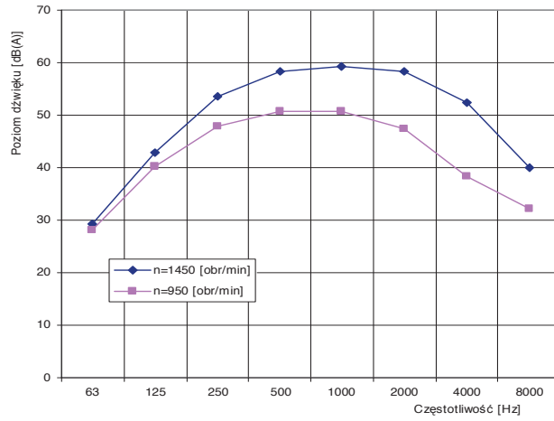
Charakterystyka akustyczna wentylatora dachowego WDC/s 25-Ex (na wlocie w odległości 1m)
