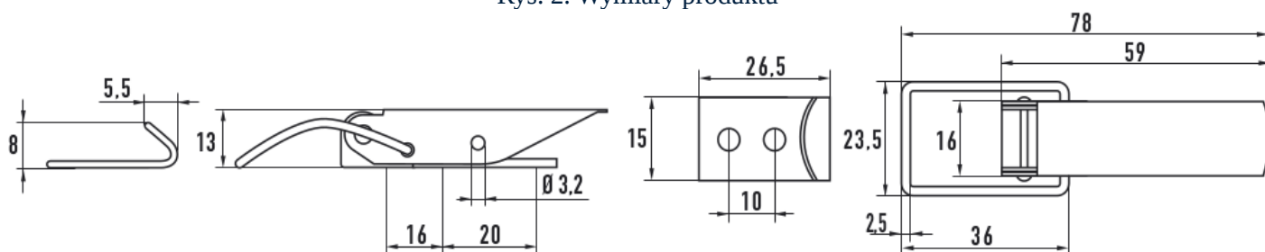
Rys. 2. Wymiary produktu
